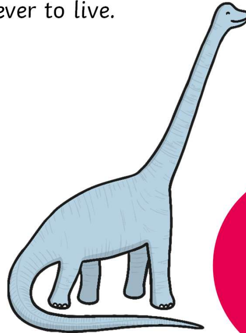
Brachiosaurus
