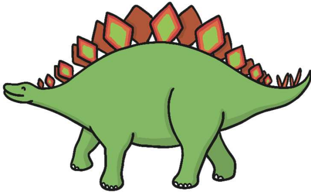
Stegosaurus
