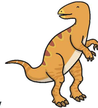
Iguanodon
