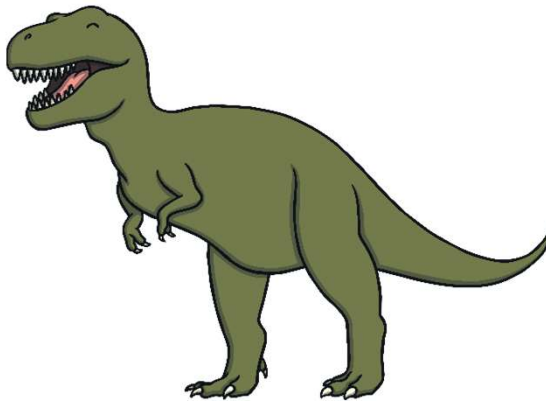
Tyrannosaurus-Rex
