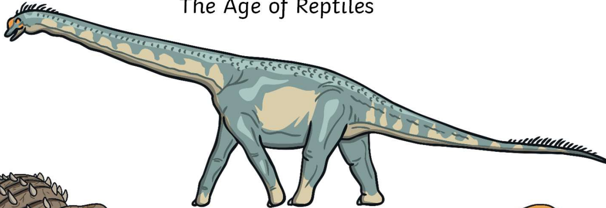
Titanosaurs
