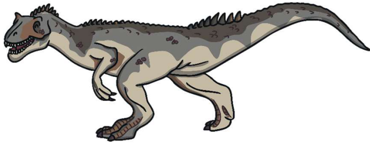
Allosaurus
