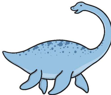
Plesiosaur
