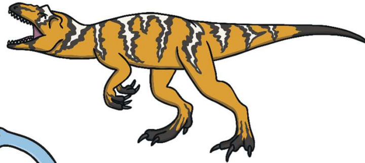
Epanterias
